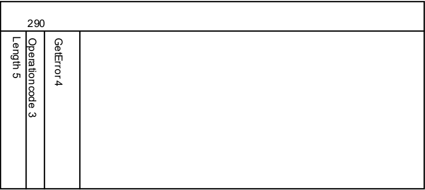
Figuur 6.17 Structuur GetMessageConfirmation
