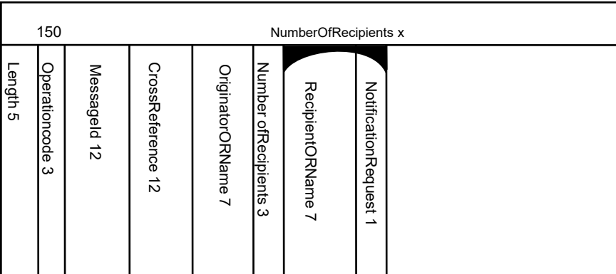
Figuur 6.7 Structuur MessageHeading
