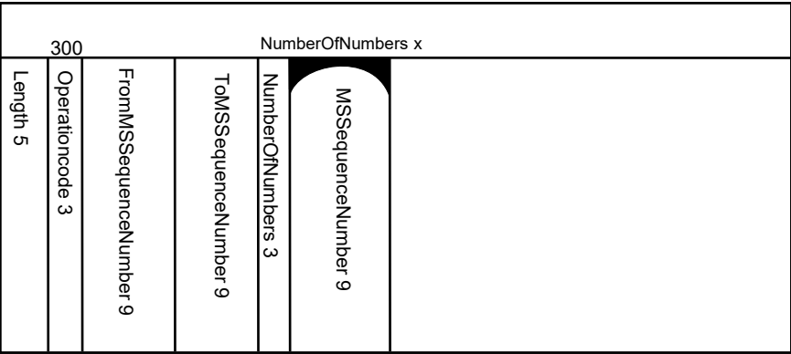
Figuur 6.18 Structuur DeleteMessages
