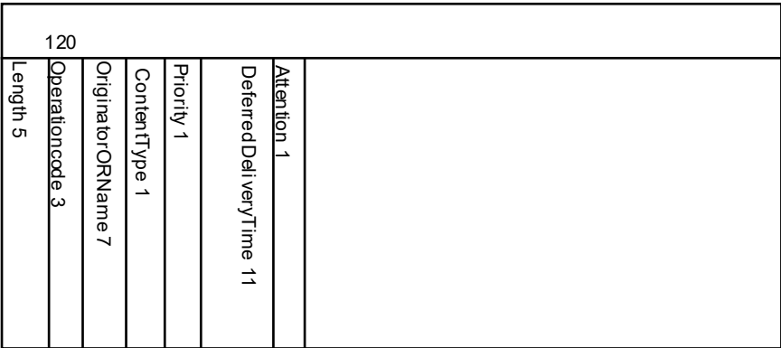
Figuur 6.6 Structuur PutEnvelope
